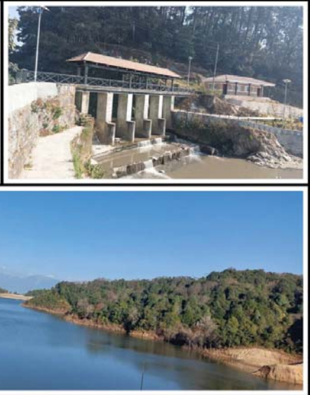
बागमती नदी (माथि) र शिवपुरीमा निर्माण सम्पन्न भएको धाप ड्याम ।
