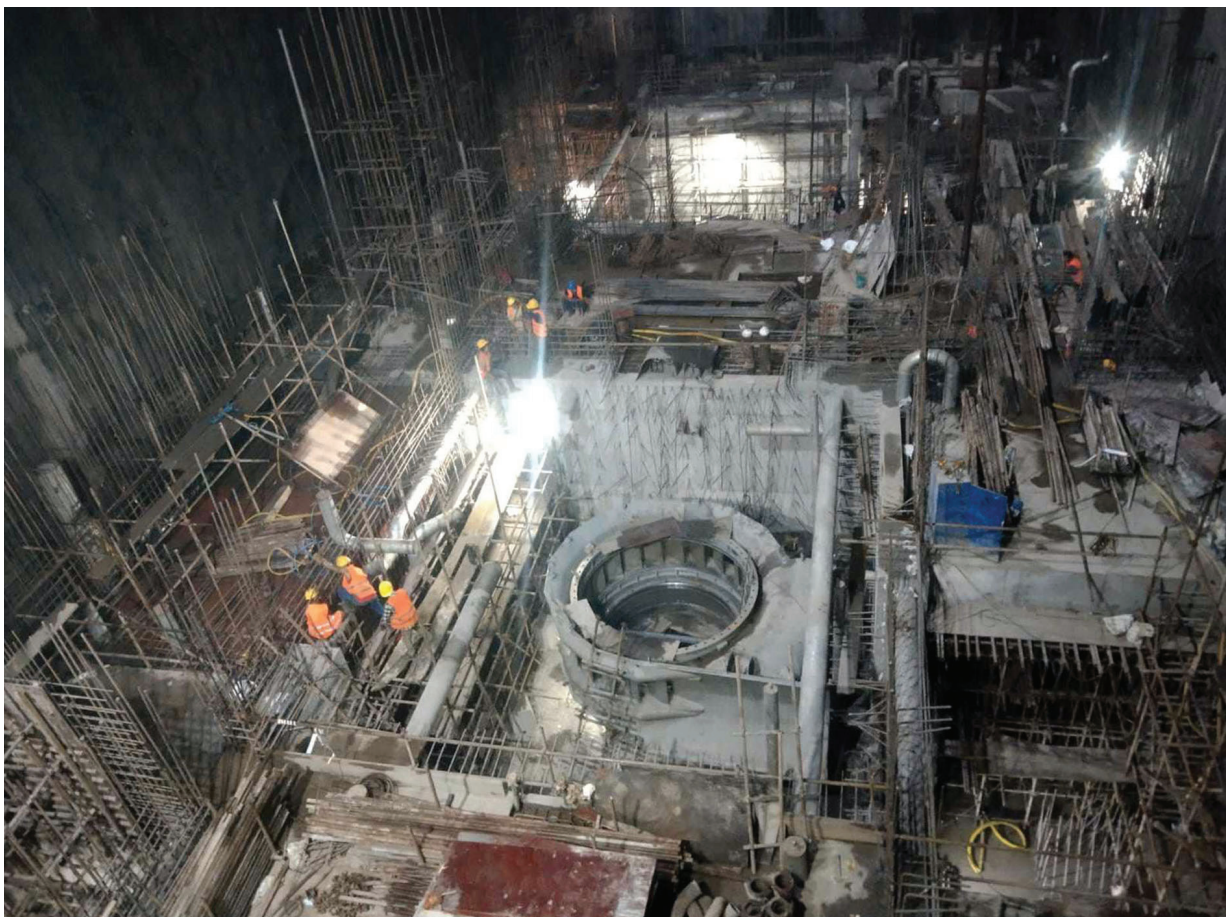
भूमिगत विद्युत्गृहमा तनहुँको ऋषिङ गाउँपालिका-१ मा निर्माणाधीन १४० मेगावाट क्षमताको तनहुँ जलविद्युत् आयोजनाको भूमिगत विद्युत्गृहमा काम धमाधम। धमाधम काम हुँदै। आयोजनाले तीन वटै प्याकेजका कामलाई तीव्रता दिएको छ। तस्विर: कृष्ण न्यौपाने/रासल
